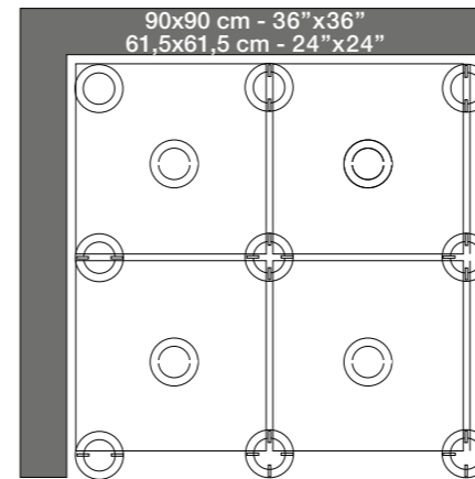
Supporti regolabili e supporti autolivellanti Adjustable supports and self-leveling supports Supports réglables et supports auto-nivelants Höhenverstellbarer Träger und Selbstnivellierender Träger
